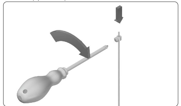
12. Auf eines der Enden der Schnurführungsschiene ein Anschlagring aufstecken und anschließend den Anschlagring durch Anziehen der Einstellschraube fixieren, um Abrutschen des Anschlagrings zu verhindern.
