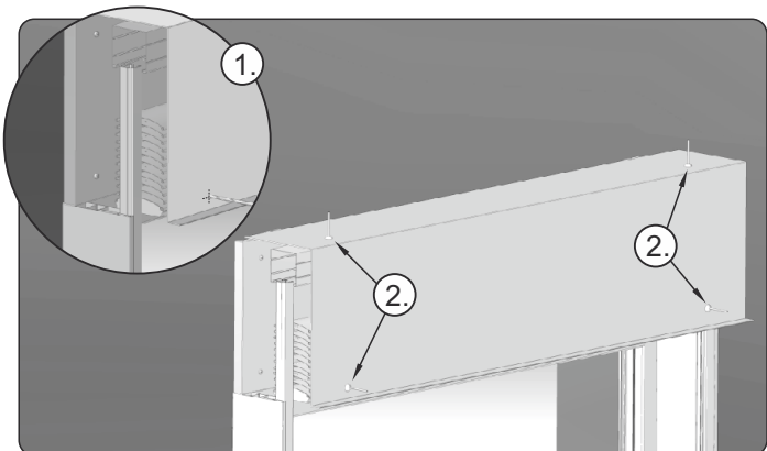
17. Die Löcher (1) in dem Schutzblech an den Stellen, an denen das Blech an den Halterungen und Verlängerungen befestigt werden soll, bohren und diese dann mit 4x8 Nieten (2) vernieten.
