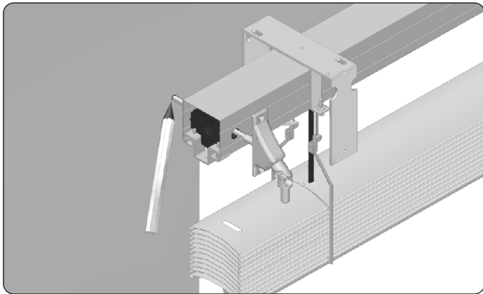
7. Bei Außenjalousien mit Handantrieb nach dem Einbau des Pakets eine Stelle für die Bohrung für Steuerungsdraht markieren.
