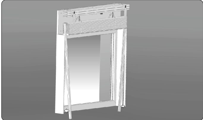
13. Die Führungsschienen in das Paket einschieben, dann die Führungsschienen von der Seite in den Adapter einschieben.
