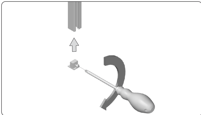
15. Die Endkappen der Führungsschienen montieren.
