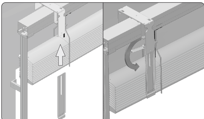
17. In die vorher eingebauten Wandhalterungen die Schutzblechverlängerungen hineinschieben und anschließend die Schutzblechverlängerungen anschrauben.
