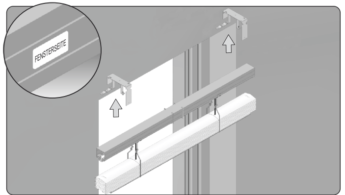
6. In die offenen Halterungen das Jalousienpaket so einbauen, damit sich der Aufkleber „FENSTERSEITE“ mit der Information über Montageseite fensterseitig befindet.
