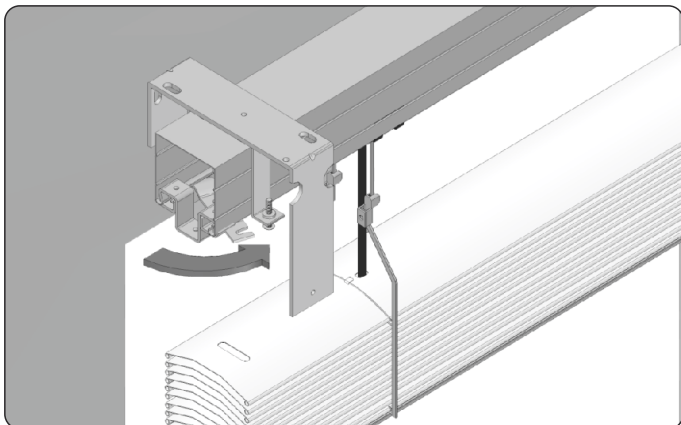
9. Halterungen der Oberschiene schließen und Schrauben anziehen.
