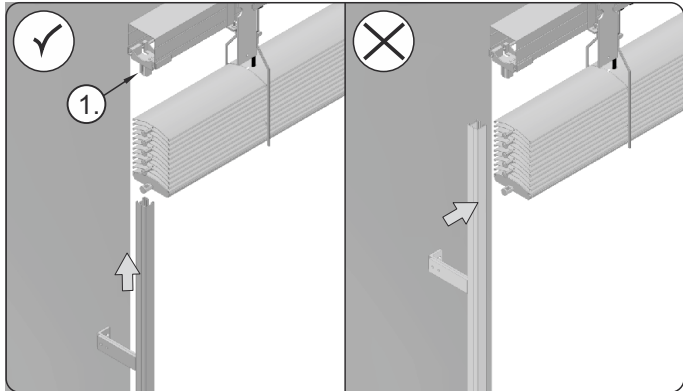
13. Die Führungsschiene mit Halterungen auf Lamellenschäfte von der Jalousienunterseite nach oben aufzustecken. Die Halterungenschäfte (1.) in den Oberteil der Führungsschienen vorsichtig einführen. Prüfen, ob die Elemente richtig zusammengebaut sind. Keine Führungsschienen der Jalousien auf Schäfte drücken – es kann zur Beschädigung der Führungsschienen führen.
