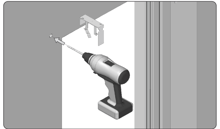
8. Paket demontieren, mit Bohrer fi 12 eine Öffnung für Steuerungsdraht im Fensterrahmen oder in der Wand (je nach der Montageart) bohren und anschließend Paket erneut in der Halterung der Oberschiene montieren.
