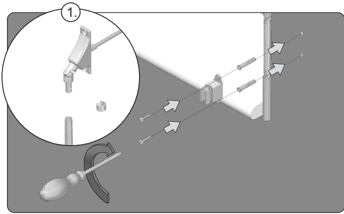
11. Den Zwischenstecker mit der gelieferten Kurbel mit Befestigungselementen verbinden (geliefert von der Firma PORTOS), wie im Abb. 1 dargestellt. Montageclip der Kurbel an die Wand mit Schrauben (Spreizdübel) anschrauben.
