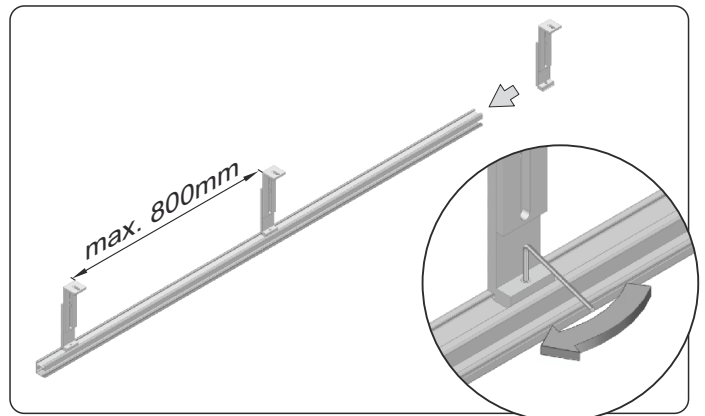
12. Die Halterung der Führungsschiene in die hintere Wand der Führungsschiene hineinschieben, durch Festziehung des Gewindestiftes fixieren. Maximaler Abstand zwischen den Halterungen soll nicht mehr als 800 mm betragen.
