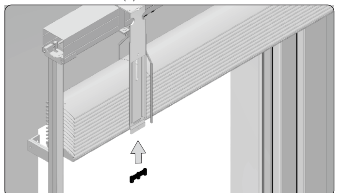
18. Auf Unterteile der Verlängerungen ein Schalldämpfelement der Verlängerung aufstecken.
