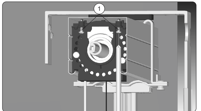
16. Nach Überprüfung der ordnungsgemäßen Funktion von Außenjalousien stellen Sie den Aufrollantrieb in einer vertikalen Fluchtlinie mit Wickelband auf und schrauben Sie anschließend die Konterschrauben (1) fest.
