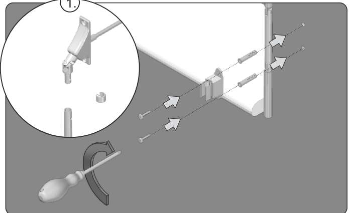
10. Den Zwischenstecker mit der gelieferten Kurbel mit Befestigungselementen verbinden (geliefert von der Firma PORTOS), wie im Abb. 1 dargestellt. Montageclip der Kurbel an die Wand mit Schrauben (Spreizdübel) anschrauben.
