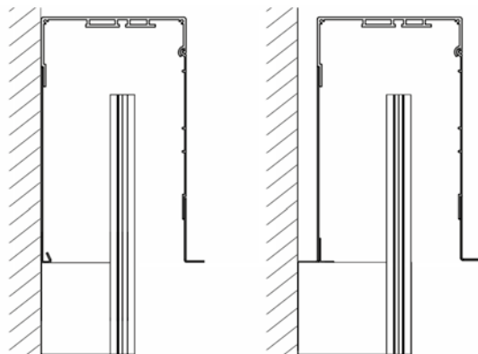
TYP A - Einbaukasten. Passende Führungsschienen F-FBR-030.
