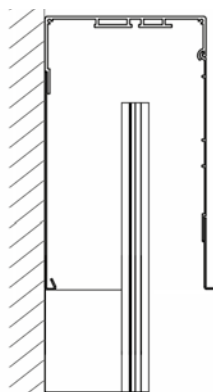
TYP A - Einbaukasten. Passende Führungsschienen F-FBR-030.
